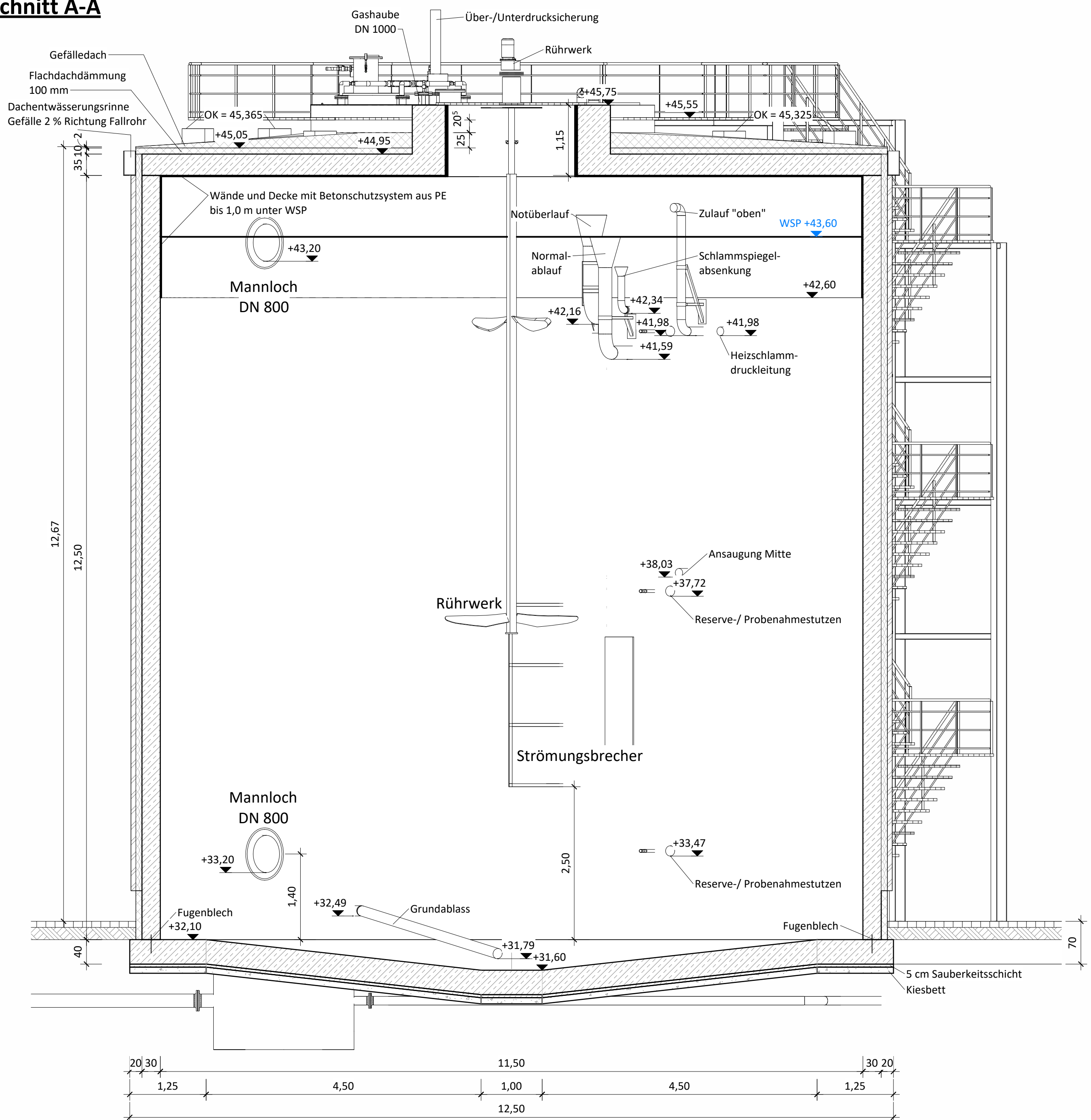
Schnitt A-A
