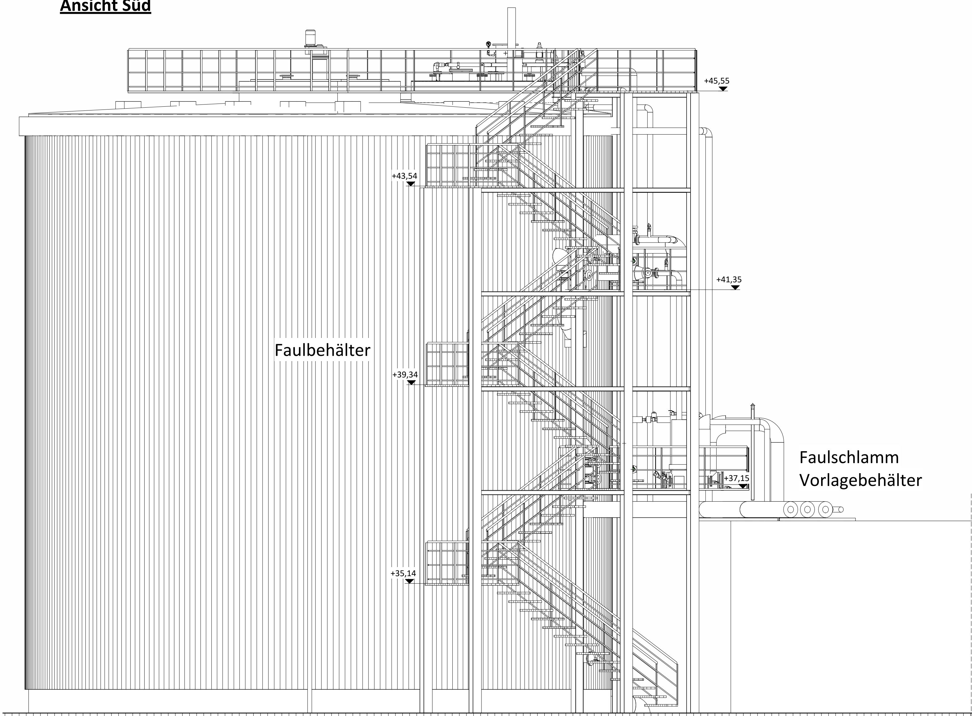
Ansicht Süd
